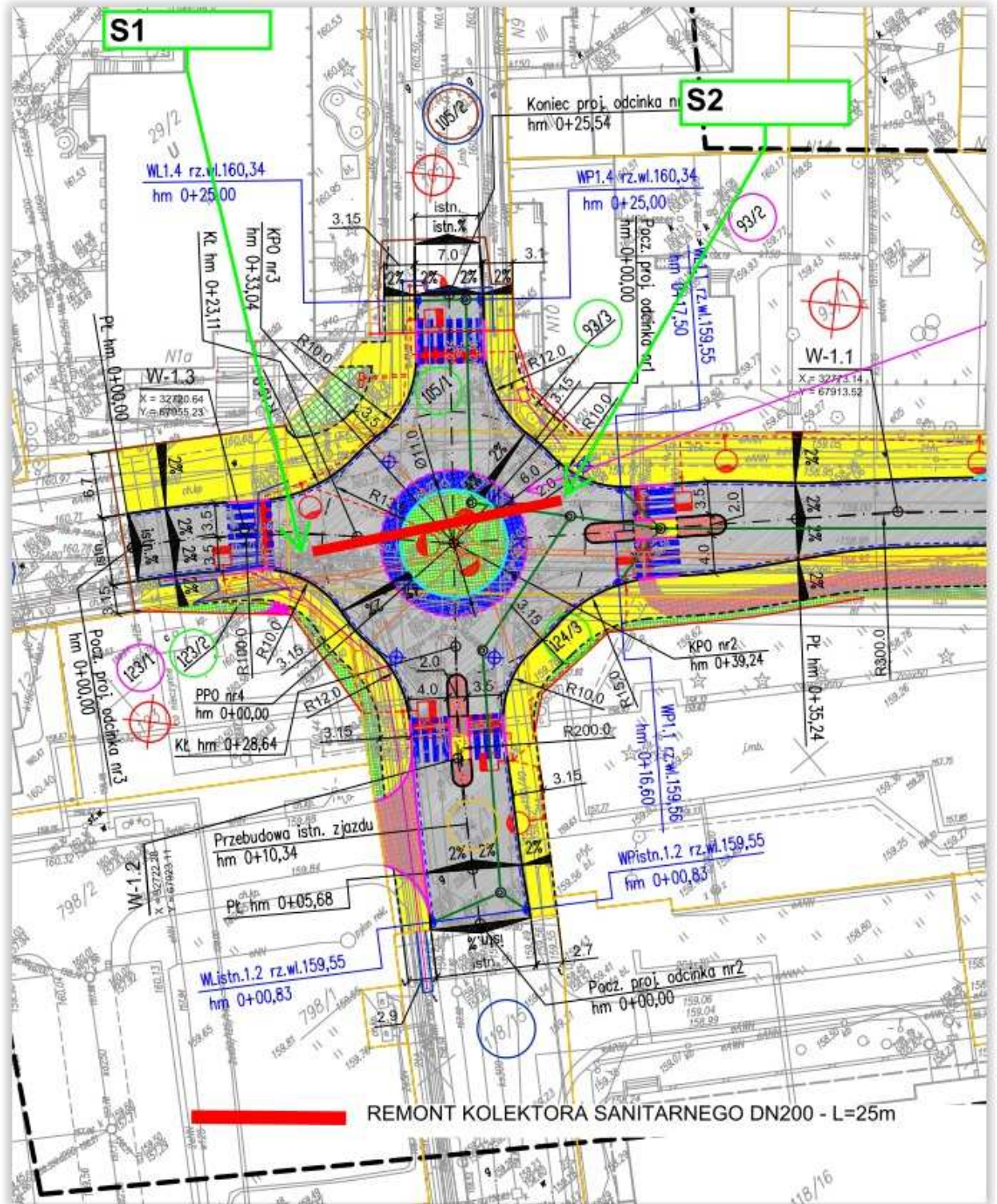
Załącznik nr 1. Plan sytuacyjny z planowanym zakresem robót ul. Artylerzystów w Żarach.
