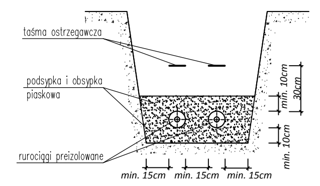
Schemat zabudowy rur preizolowanych Delta PEX Heat UNO w wykopie
