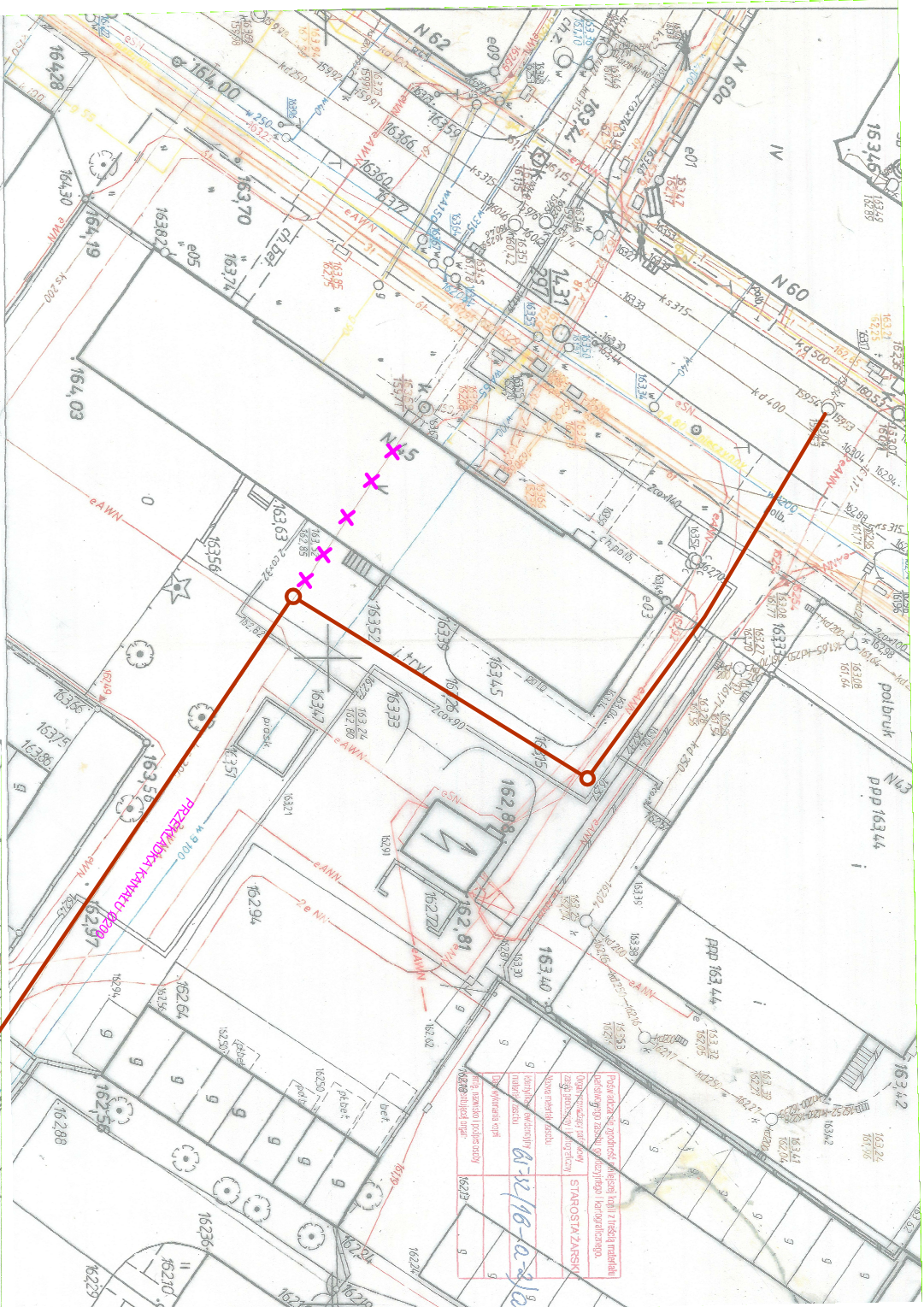
— Kanalizacja Ø200, L=109m,
